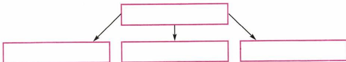
Состав гранита
